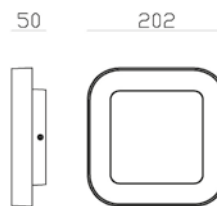
Wandleuchte - Quadratisch
