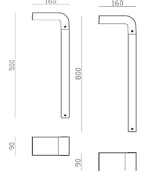
L-förmige Pollerleuchte
