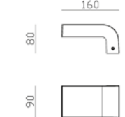
L-förmige Wandleuchte
