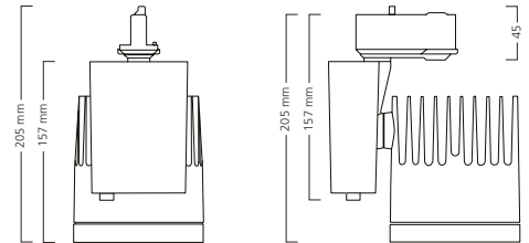
Abmessungen (mm)
